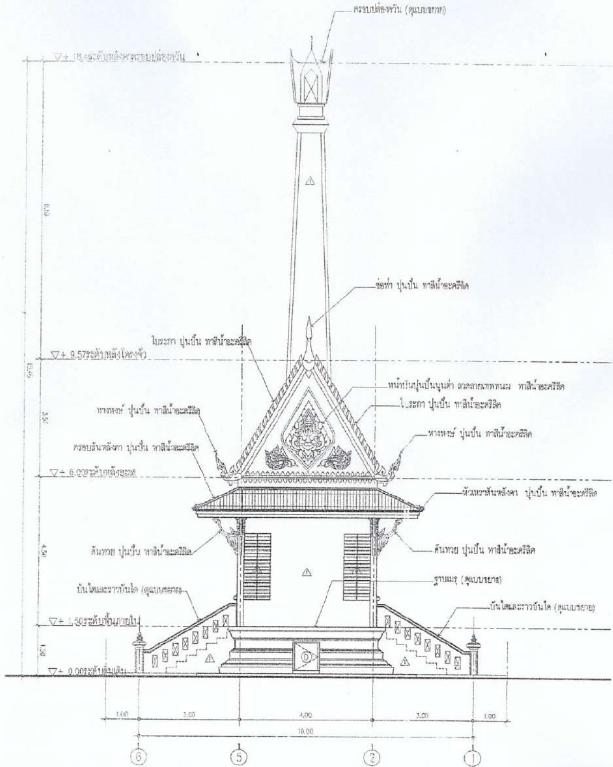
แบบแสดง รูปด้าน 3. ขนาด 1:75
