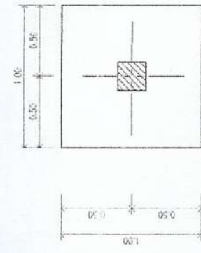
แบบขยาย ฐานเสา F3 SCALE 1:25
