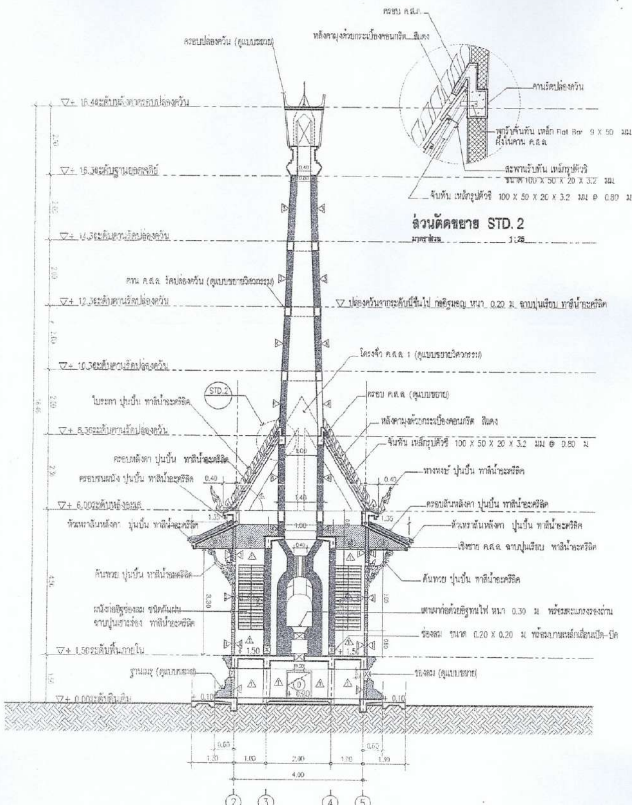
แบบแสดง รูปตัด C. มาตรฐาน 1:75
