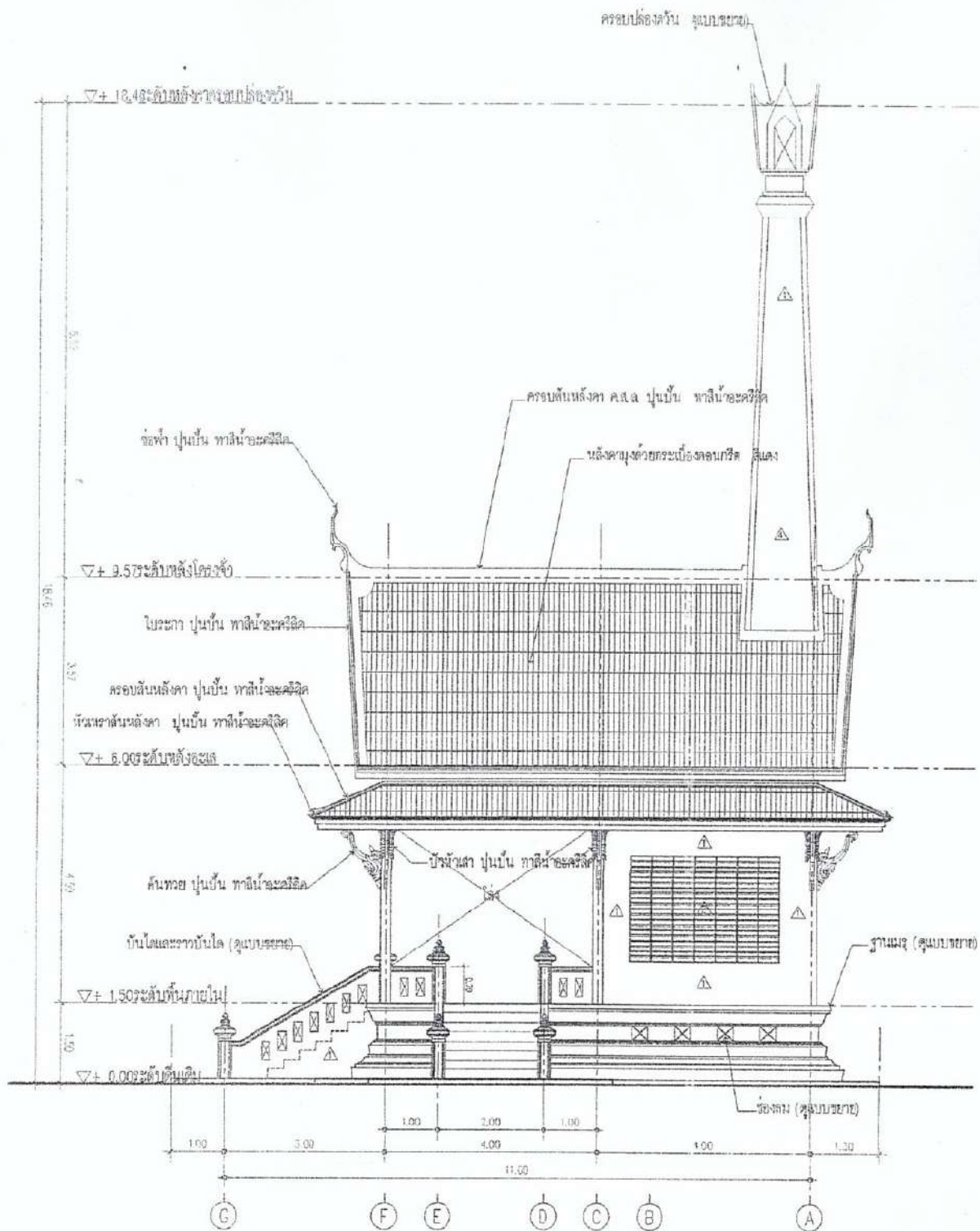
แบบแสดง รูปด้าน 4 ขนาดย่อ 1:75
